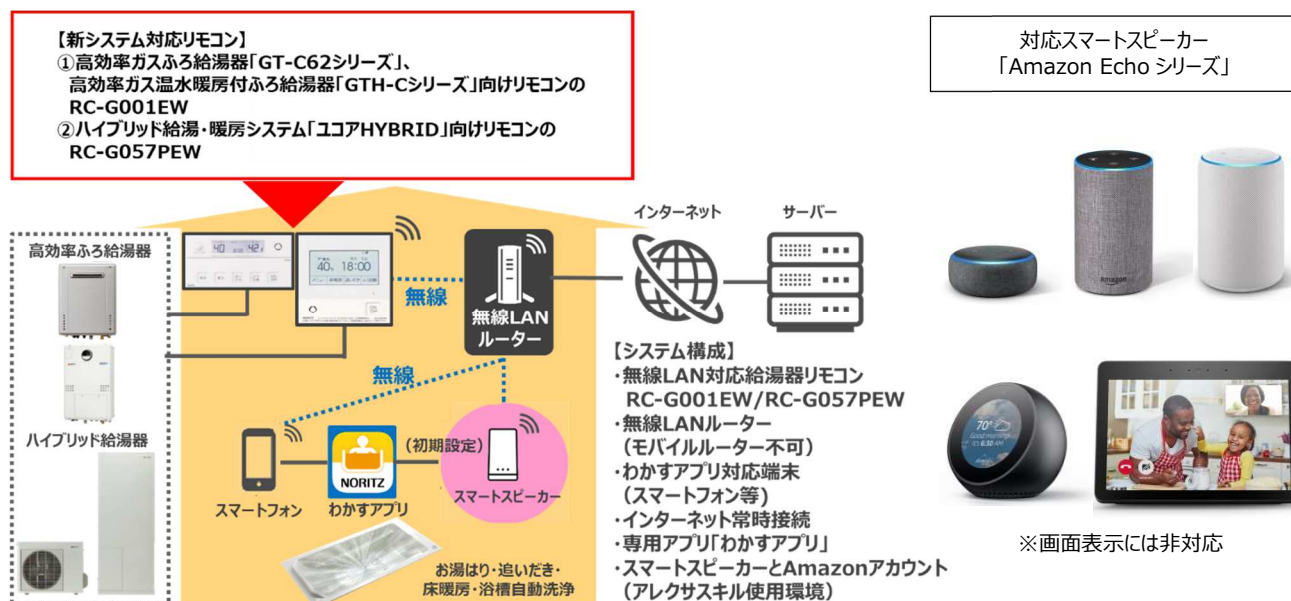
システム構成図
